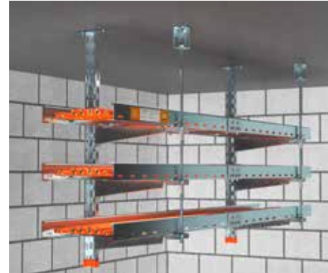
Deckenmontage mit Hängestiel und Ausleger
